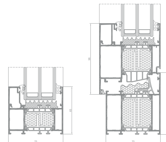
Vue en coupe à travers une fenêtre GN 75 (GN 011)
