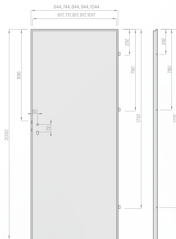
vantail avec paumelles visibles
