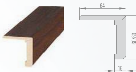
CORNIÈRE AVEC AILE PROLONGÉE POUR DORMANT RÉGLABLE chambranle 6 cm / chambranle 8 cm
