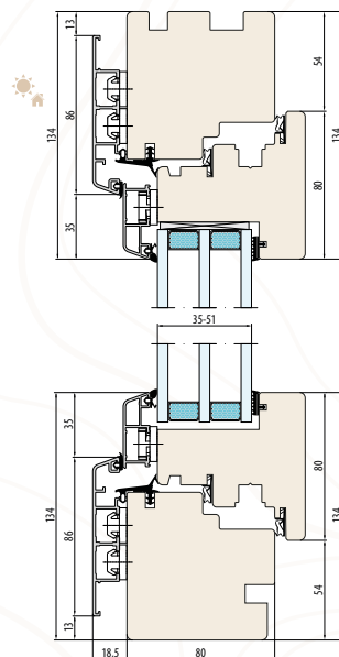
SYSTÈME NATURO 80 ALU GEMINI CLASSIC découpe pour l'appui de fenêtre intérieur
