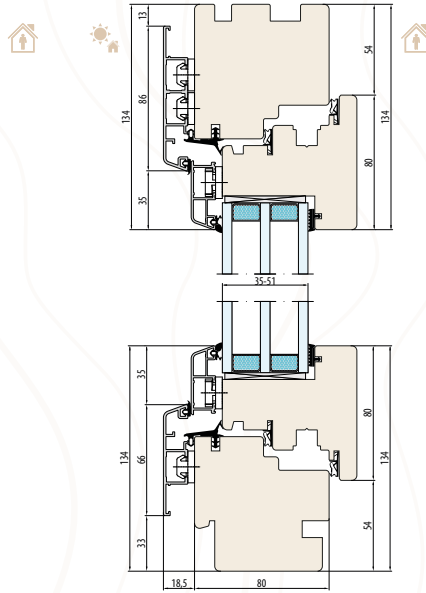
SYSTÈME NATURO 80 ALU GEMINI CLASSIC découpe pour l'appui de fenêtre intérieur et extérieur
