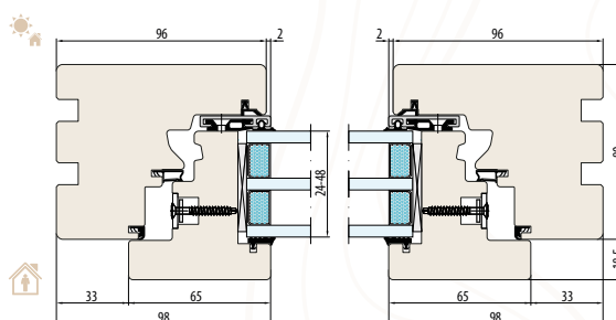
SYSTÈME ESPERIA LIFE 80 SECTION HORIZONTALE B-B
