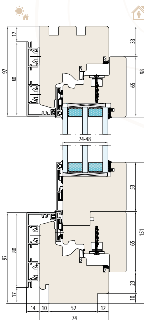
SYSTÈME ESPERIA LIFE 74 ALU portes-fenêtres à un vantail avec seuil relevé
