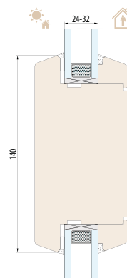
SYSTÈME NATURO 68 meneau structurel 140 mm
