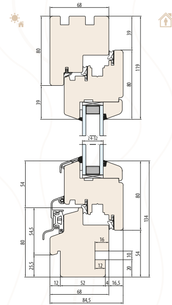
SYSTÈME NATURO 68 découpe pour l'appui de fenêtre intérieur et extérieur
