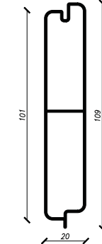
Panneau planchette
